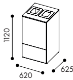
W3113 Dörr ovan till för 2x60 l kärl och lādutdrag undertill *
