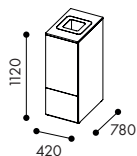
W3214 Dörr ovan till för 1x60 l i kärl och lådudrag undertill **
