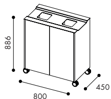
W93- Dubbel på hjul
