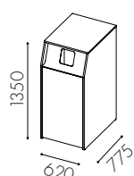
W3518 Hel dörr för rullkär 190 liter *
