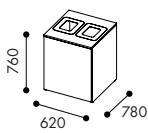
W3216 Låg modul med hel dörr för 2x60 l i kärl
