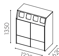
W3517 Dörr ovan till för 2x60 l kär och låd utdrag undertill **
