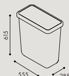
W0015 Kärl 60 liter
