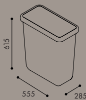
W0115 Kärl 60 liter Ett kärl ryms i varje utdragslåda
