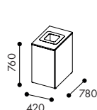
W3217 Låg modul med hel dörr för 1x60 l i kärl
