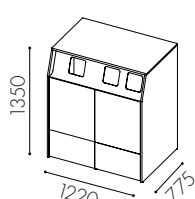
W3524 Dörr ovan till för 90 l kär i enkelt in kast, 2x60 i dubbelt in kast och låd utdrag undertill **
