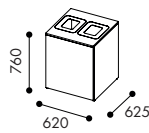
W3116 Låg modul med hel dörr för 2x60 l kärl
