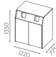
W3521 Hela dörrar för rullkär 190 liter *
