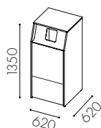
W3511 Dörr ovan till för 90 l kär och låd utdrag undertill **
