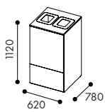
W3213 Dörr ovan till för 2x60 l i kärl och lådudrag undertill *
