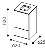
W3112 Dörr ovan till för 1x90 l kärl och lādutdrag undertill *
