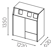
W3515 Hel dörr till vänster för rullkär 140 l *, dörr ovan till för 2x60 kär och låd utdrag undertill till höger **
