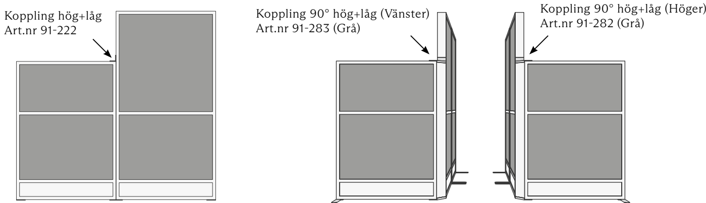
EXEMPEL (Hög + låg kopplingar)
