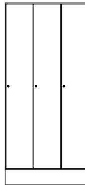
KLT90 898x1936x570
