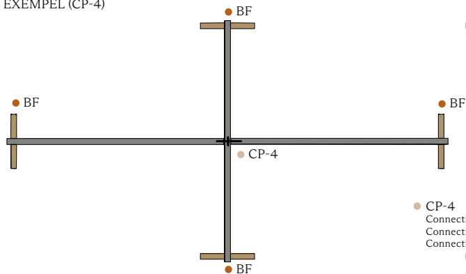
EXEMPEL (CP-4)
