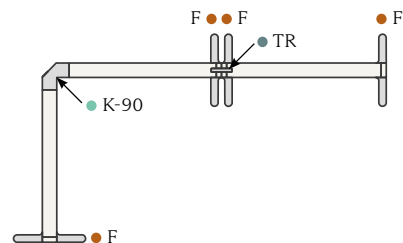
EXEMPEL (Koppling 90°)
