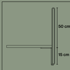
Frontmonterat beslag artikelnr. 3132
