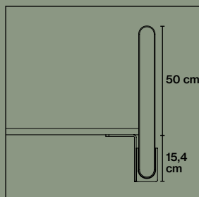
Frontmonterat beslag artikelnr. 5032
