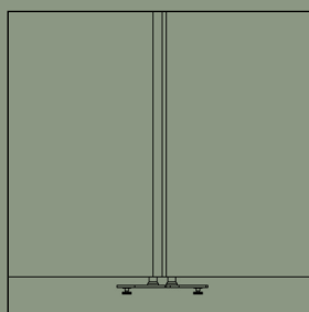
Justerbar samlefot artikelnr. 5125
