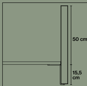
Frontmonterat beslag artikelnr. 5132
