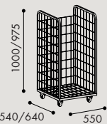
W0101 Vagn för kartonger M W0103 Sidor till vagn M W0102 Vagn för kartonger L W0104 Sidor till vagn L
