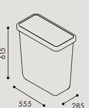
W0015 Kärl 60 liter
