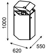
W6521 Arch för befintlig stolpe för utomhusbruk Avfallsvolym: 210 liter (3x70L)
