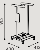
W0089 Säckhållare 125 liter
