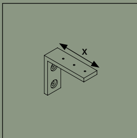
Väggbeslag artikelnr. 311X**
