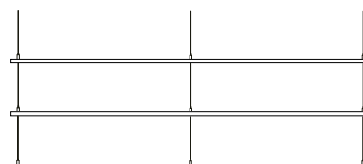
3 st rundstavar 3100 med vajerkit till tak samt vajerkit mellan rundstavar
