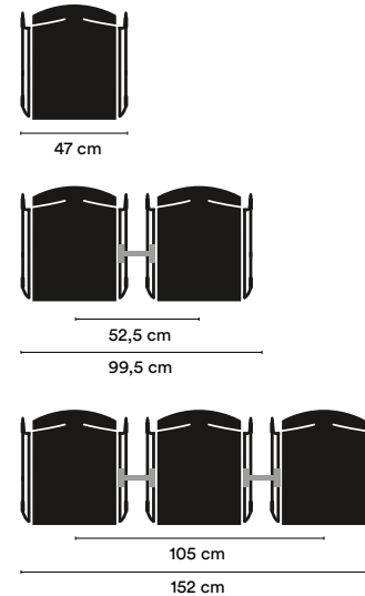
Chairik 128XL med länkanordning CH192, CH193 & CH199*
