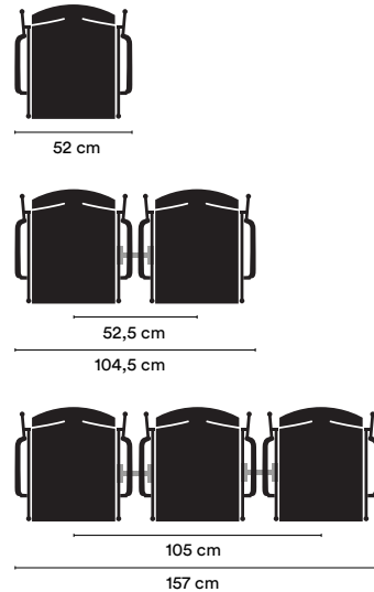
Chairik 127XL med länkanordning CH192, CH193 & CH199*
