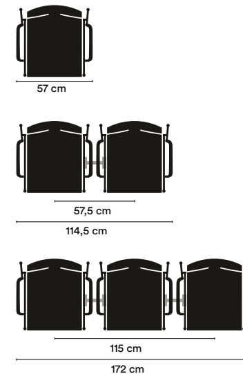
Chairik 123XL & 129XL med länkanordning CH194 & CH195
