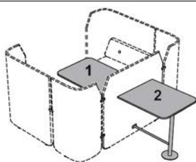
Bord med pelare för bordshöjd 900 mm För sida 1 och/eller sida 2.
