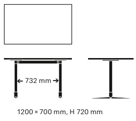
1200 x 700 mm, H 720 mm
