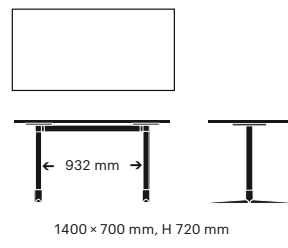
1400 x 700 mm, H 720 mm
