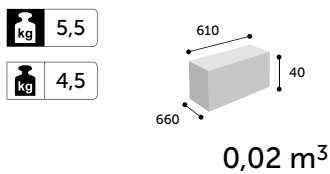
frame CS30
