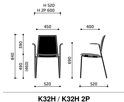
K32H / K32H 2P
