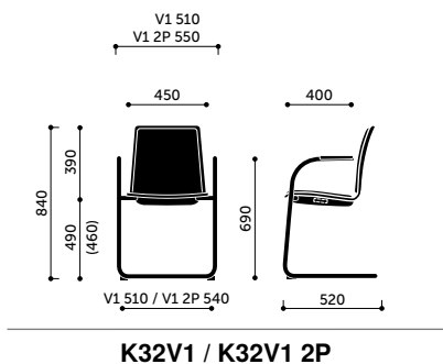
K32V1 / K32V1 2P
