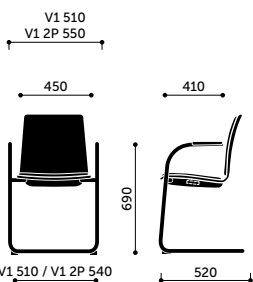
K22V1 / K22V1 2P
