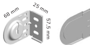
Standardbeslag Art.nr. R38987-88
