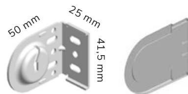
Standardbeslag Art.nr. R28155-57
