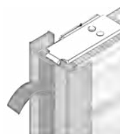
(A1) U-list med tejp och vinkel. Till modell 3242 levereras vinkel tillsammans med wirefot. Sidolisten kan också monteras på glas.
