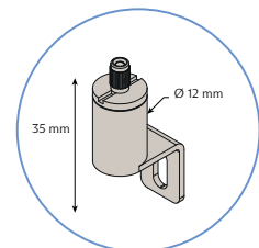
Vajerhållare för väggmontering
