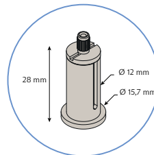
Vajerhållare för golv-/karmmontering
