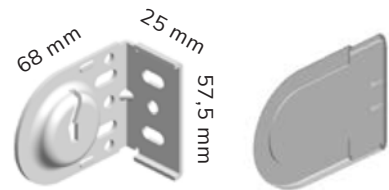
Standardbeslag Art.nr. R38987-88
