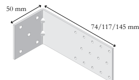
Vinkel, 10/12,5 cm 35/50/70 mm
