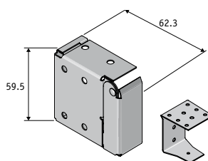
Ändbeslag, special - U-beslag för mittplacering
