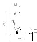
Skylight sidolist
