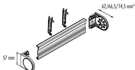
Modell 20 Monteringsprofil
