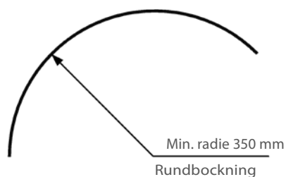
Rundbockning
