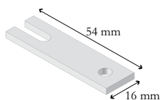
Distans till takmontering - Sidodrag/motor (standardbeslag)
