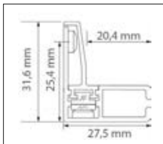
Sidolist, typ 2/3.
