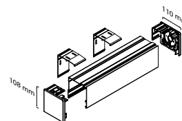
Modell XXL-270/290 Heavy Duty Kassett Sidokanaler som tillval
