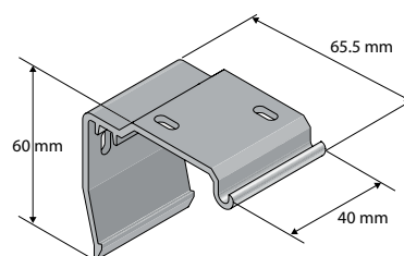
Design XL, clipsbeslag
