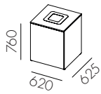
W3115 Låg modul med hel dörr för 1x90 l kärl
