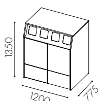
W3525 Dörr ovan till för 2x60 l kär och låd utdrag undertill **
