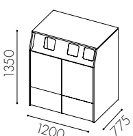
W3524 Dörr ovan till för 90 l kär i enkelt inkast, 2x60 i dubbelt inkast och låd utdrag undertill **
