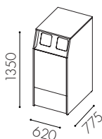
W3520 Dörr ovan till för 2x60 kär och låd utdrag undertill **
