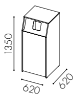
W3510 Hel dörr för rullkär 140 liter *
