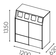
W3517 Dörr ovan till för 2x60 l kär och lådutdrag undertill **
