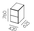
W3121 2-låds modul * *
