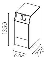
W3519 Dörr ovan till för 90 l kär och lådutdrag undertill **
