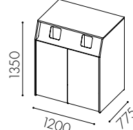
W3521 Hela dörrar för rullkär 190 liter *
